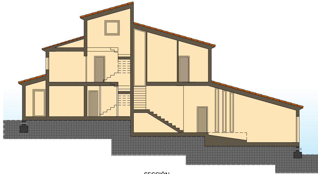
SECCIÓN
