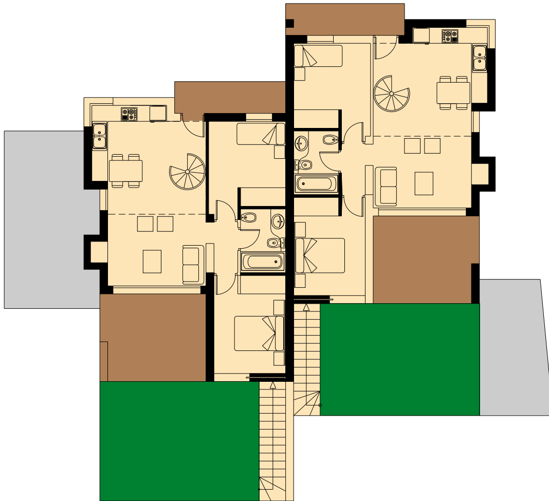
PLANTA BAJA
